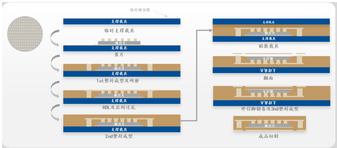
无框架、无基板封装结构示意图
